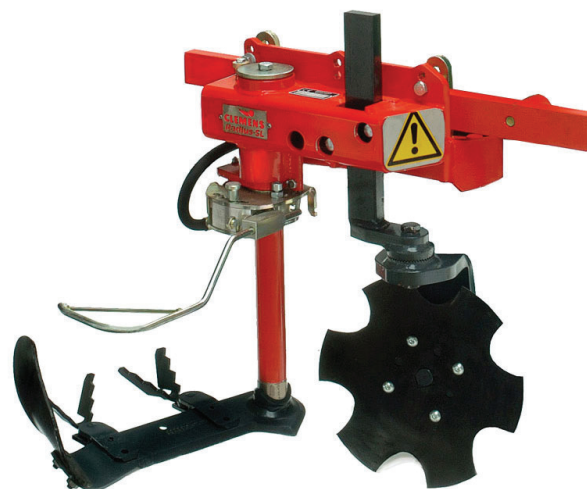
Slika 22. Mehaničko suzbijanje korova obradom tla u zaštitnom prostoru
